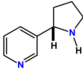
nicotine
